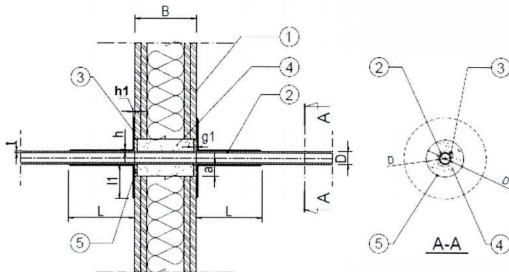
Rys. C12. Uszczelnienie przejść instalacyjnych małych kabli w korytku kablowym ( \phi \leq 13 \text{ mm} ) przez ścianę podatną lub sztywną o grubości t > 100 \text{ mm} , wykonane za pomocą Flame Cabel Farba.
