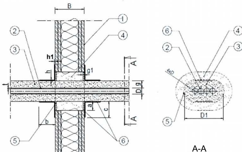
Rys. C3. Uszczelnienie przejść instalacyjnych rur metalowych w wiązce (max. 4 rur w wiązce) przez ścianę podatną lub sztywną, wykonane za pomocą Flame Cabel Pasta A (z ciągłą izolacją z wełny mineralnej).
