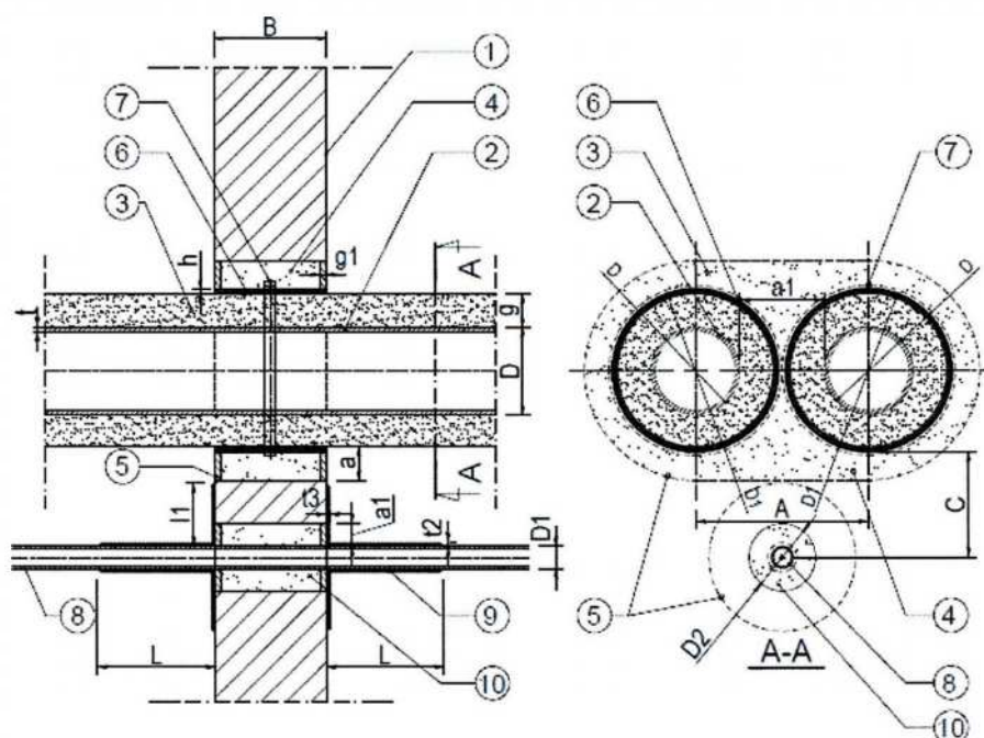
Rys. C13. Uszczelnienie przejść instalacyjnych rur metalowych za pomocą Multitube Wrap o szerokości 100 mm i grubości 4,8 mm z dodatkowym pojedynczym kablem (o \varnothing 13 mm) wykonane za pomocą Flame Cabel Farba przez strop sztywny (z ciągłą izolacją z elastycznej pianki elastomerowej (FEF)).
